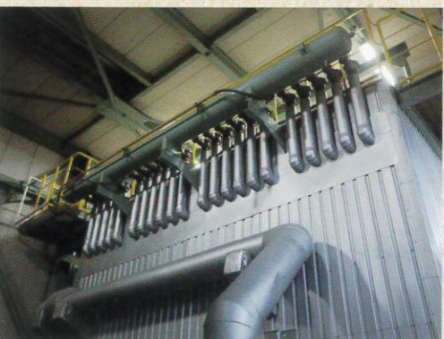
⑤ バグフィルタ
